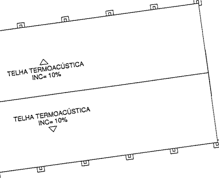
Planta Cobertura 1:100
